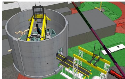
Simulation de mécanisme complexes
