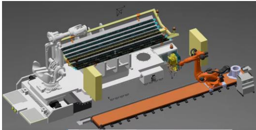
Perçage & Rivetage
